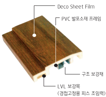
PVC 발포 일체형 프레임
